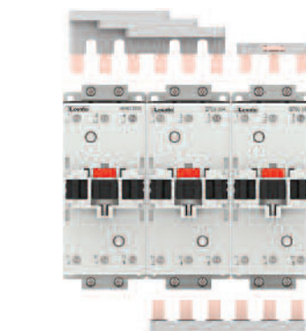
Пускатель "звезда-треугольник"
