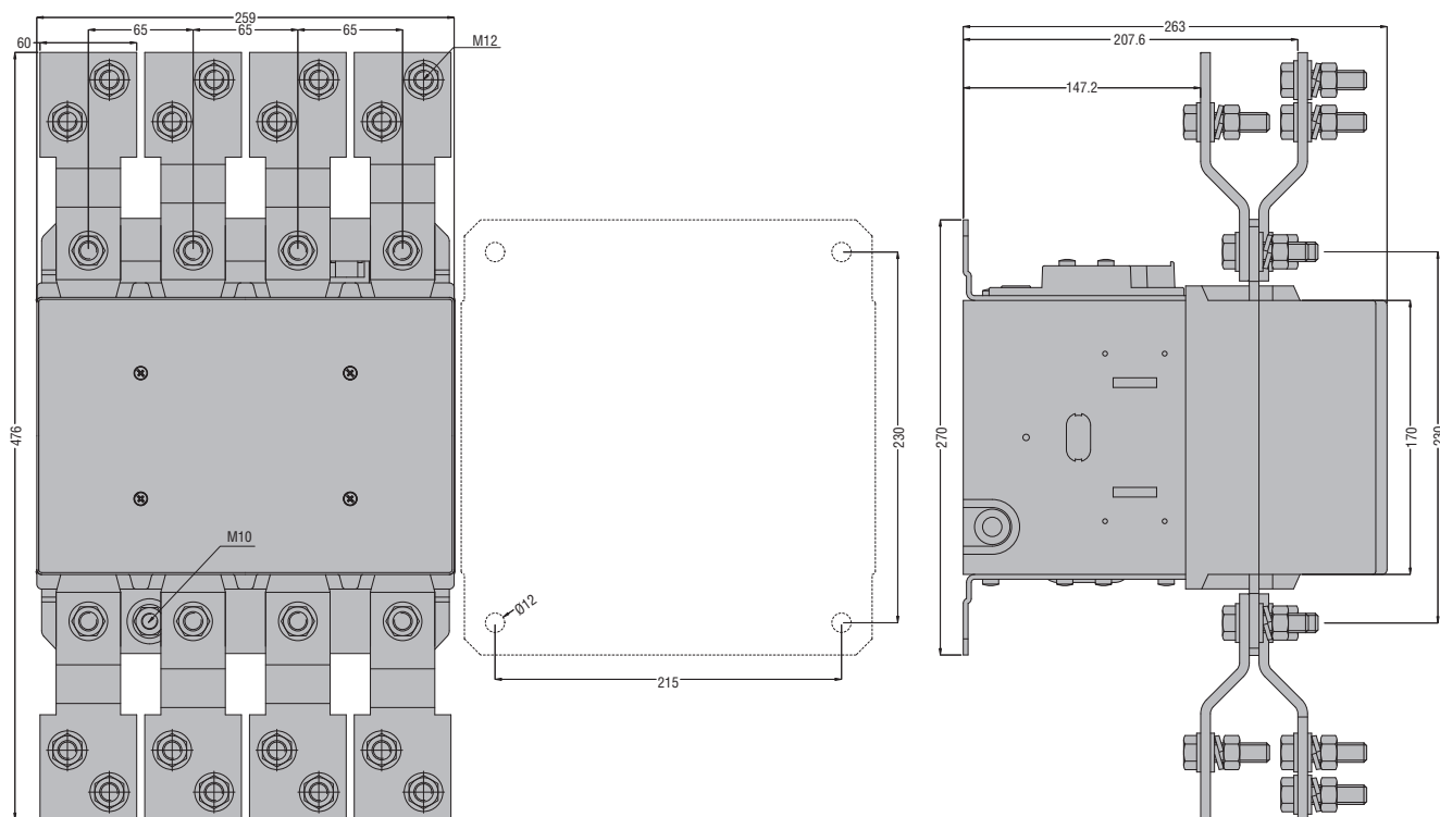
B63010004 четырехполюсные
